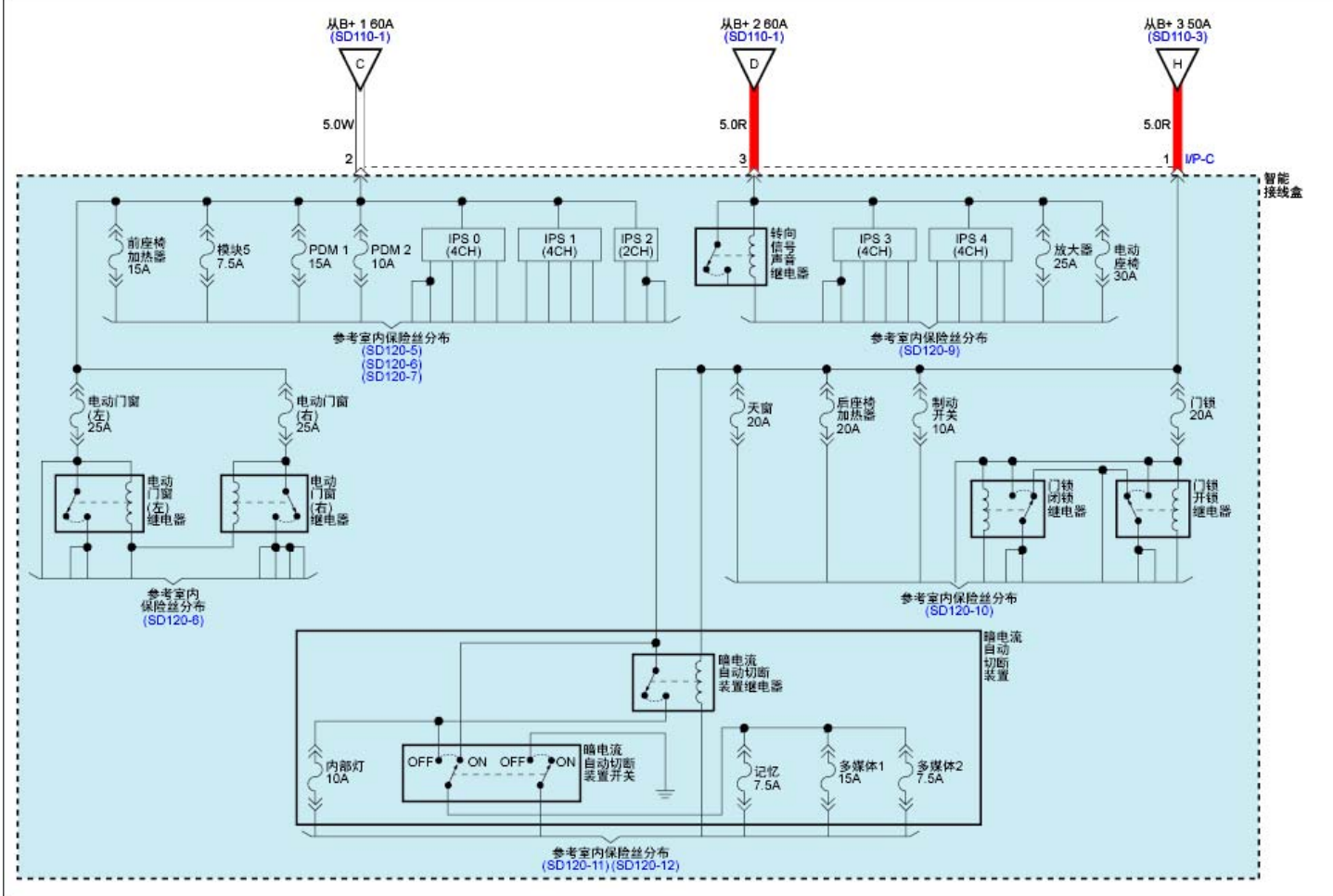
电源分布(8)
